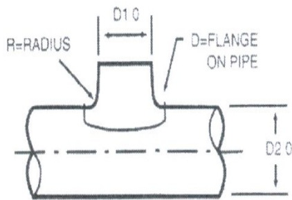
DC - TAP 45° OR 90° TAP
